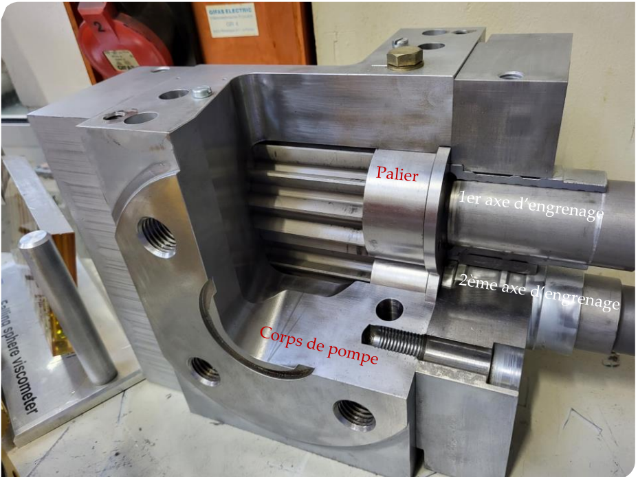
Vue d'une pompe coupée avec les 2 arbres et l'engrenage qui entraîne le polymère
